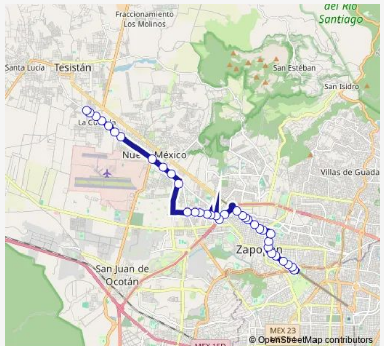
C136 — Valle de la Providencia - Plaza Patria
