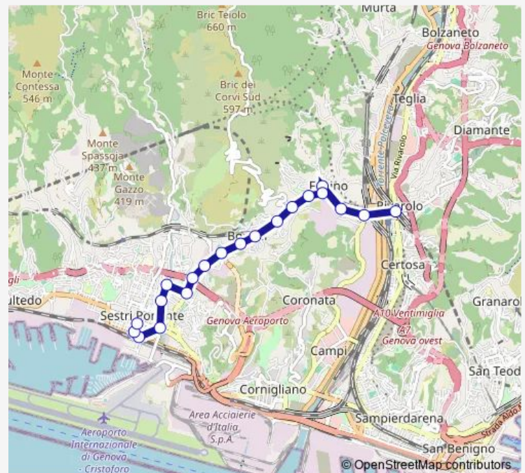
653 — Travi-Consigliere-P.zza Baracca-Rivarolo
