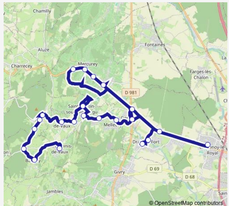
Dc4 — Vers Condorcet
