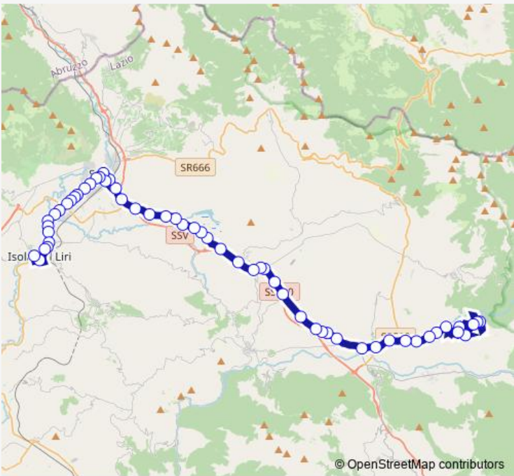
So337d — Picinisco - Isola del Liri # So337d
